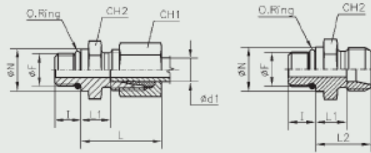
Filettatura: UNF/UN Thread: UNF/UN
